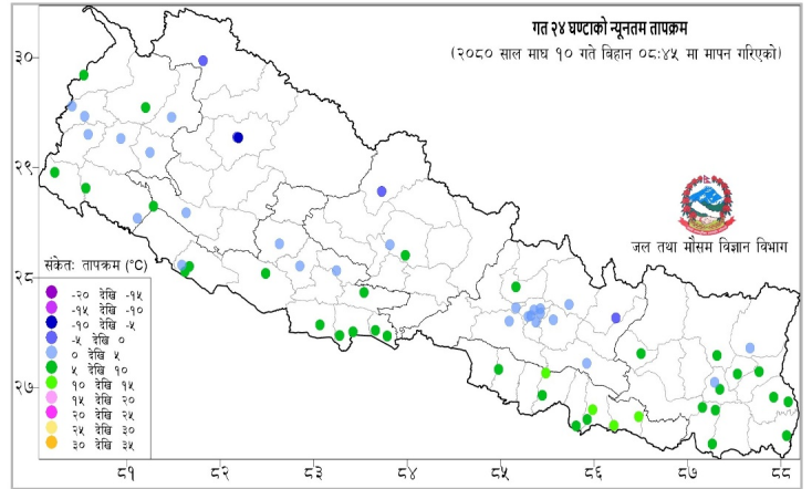
नक्सा ३: माघ ०९ गते बिहान ०८:४५ बजे देखि माघ १० गते बिहान ०८:४५ बजे सम्मको २४ घण्टाको न्यूनतम तापक्रम (डिग्री सेल्सियस)
