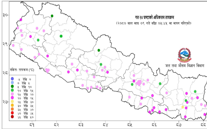
नक्सा २: माघ ०८ गते साँझ ०५:४५ बजे देखि माघ ०९ गते साँझ ०५:४५ बजे सम्मको २४ घण्टाको अधिकतम तापक्रम (डिग्री सेल्सियस)
