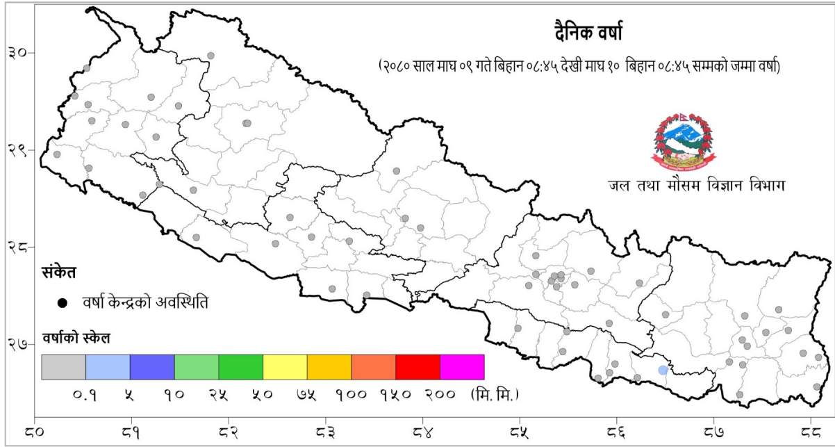
नक्सा १: माघ ०९ गते बिहान ०८:४५ बजे देखि माघ १० गते बिहान ०८:४५ बजे सम्मको २४ घण्टाको वर्षा (मि. मि.)
