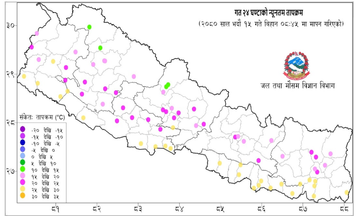
नक्सा ३: भदौ १४ गते बिहान ०८:४५ बजे देखि भदौ १५ गते बिहान ०८:४५ बजे सम्मको २४ घण्टाको न्यूनतम तापक्रम (डिग्री सेल्सियस)
