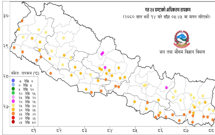
नक्सा २: भदौ १३ गते साँझ ०५:४५ बजे देखि भदौ १४ गते साँझ ०५:४५ बजे सम्मको २४ घण्टाको अधिकतम तापक्रम (डिग्री सेल्सियस)
