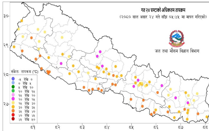
नक्सा २: असार २३ गते साँझ ०५:४५ बजे देखि असार २४ गते साँझ ०५:४५ बजे सम्मको २४ घण्टाको अधिकतम तापक्रम (डिग्री सेल्सियस)
