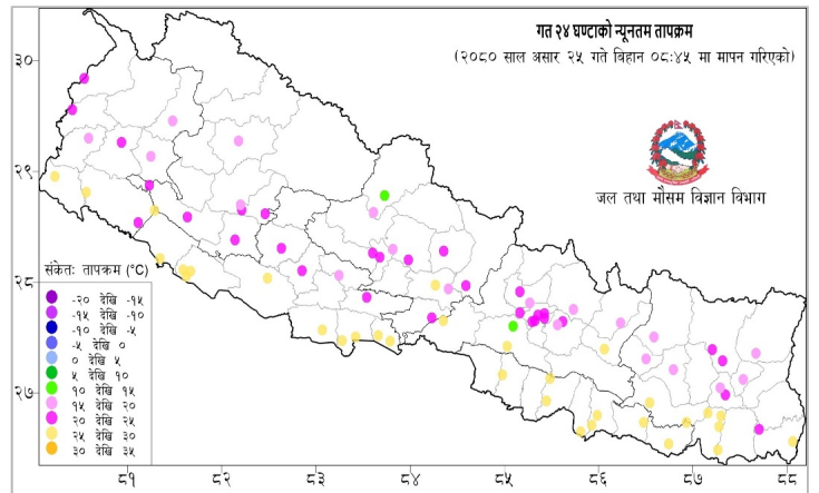
नक्सा ३: असार २४ गते बिहान ०८:४५ बजे देखि असार २५ गते बिहान ०८:४५ बजे सम्मको २४ घण्टाको न्यूनतम तापक्रम (डिग्री सेल्सियस)
