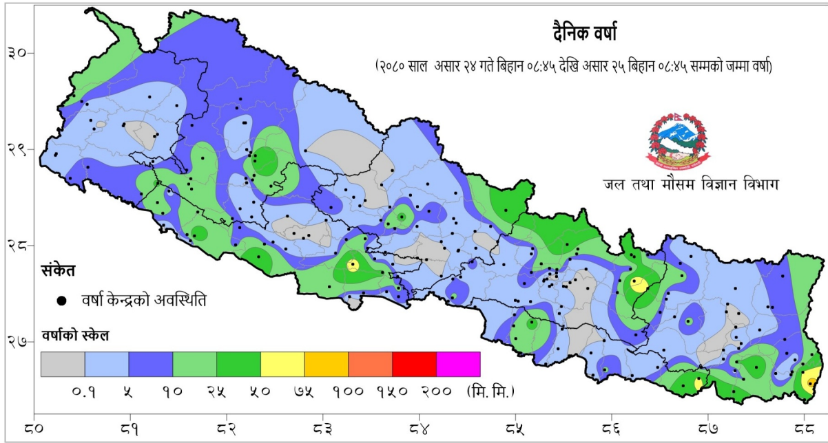
नक्सा १: असार २४ गते बिहान ०८:४५ बजे देखि असार २५ गते बिहान ०८:४५ बजे सम्मको २४ घण्टाको वर्षा (मि. मि.)
