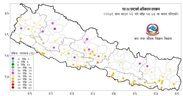
नक्सा ३: साउन ०५ गते साँझ ०५:४५ बजे देखि साउन ०६ गते साँझ ०५:४५ बजे सम्मको २४ घण्टाको अधिकतम तापक्रम (डिग्री सेल्सियस)
