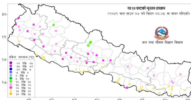
नक्सा २: साउन ०६ गते बिहान ०८:४५ बजे देखि साउन ०७ गते बिहान ०८:४५ बजे सम्मको २४ घण्टाको न्यूनतम तापक्रम (डिग्री सेल्सियस)
