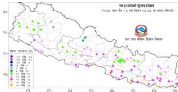
नक्सा २: चैत २२ गते बिहान ०८:४५ बजे देखि चैत २३ गते बिहान ०८:४५ बजे सम्मको २४ घण्टाको न्यूनतम तापक्रम (डिग्री सेल्सियस)
