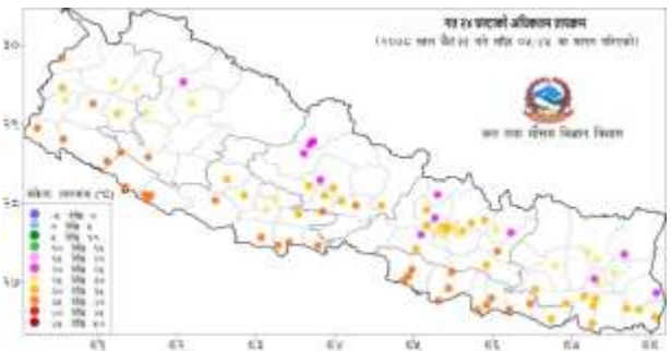
नक्सा ३: चैत २१ गते साँझ ०९:४५ बजे देखि चैत २२ गते साँझ ०९:४५ बजे सम्मको २४ घण्टाको अधिकतम तापक्रम (डिग्री सेल्सियस)
