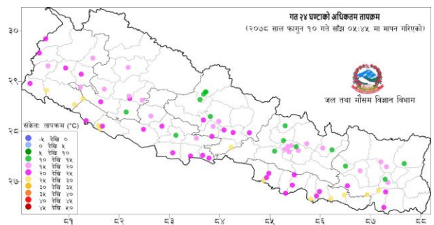
नक्सा ३: फागुन ०९ गते साँझ ०५:४५ बजे देखि फागुन १० गते साँझ ०५:४५ बजे सम्मको २४ घण्टाको अधिकतम तापक्रम (डिग्री सेल्सियस)
