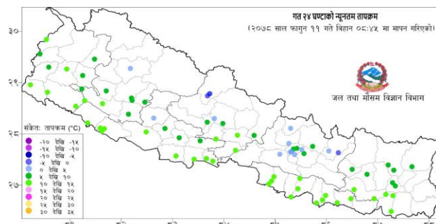
नक्सा २: फागुन १० गते बिहान ०८:४५ बजे देखि फागुन ११ गते बिहान ०८:४५ बजे सम्मको २४ घण्टाको न्यूनतम तापक्रम (डिग्री सेल्सियस)
