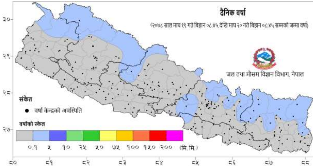
नक्सा १: माघ १९ गते बिहान ०८:४५ बजे देखि माघ २० गते बिहान ०८:४५ बजे सम्मको २४ घण्टाको वर्षा (मि. मि.)
