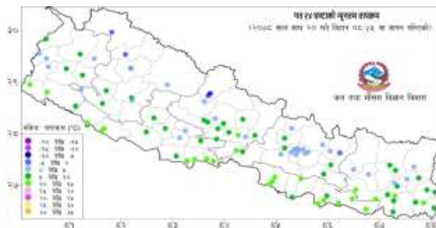
नक्सा २: माघ १९ गते बिहान ०८:४५ बजे देखि माघ २० गते बिहान ०८:४५ बजे सम्मको २४ घण्टाको न्यूनतम तापक्रम (डिग्री सेल्सियस)
