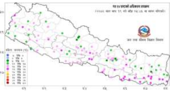
नक्सा ३: माघ १९ गते साँझ ०५:४५ बजे देखि माघ २० गते साँझ ०५:४५ बजे सम्मको २४ घण्टाको अधिकतम तापक्रम (डिग्री सेल्सियस)
