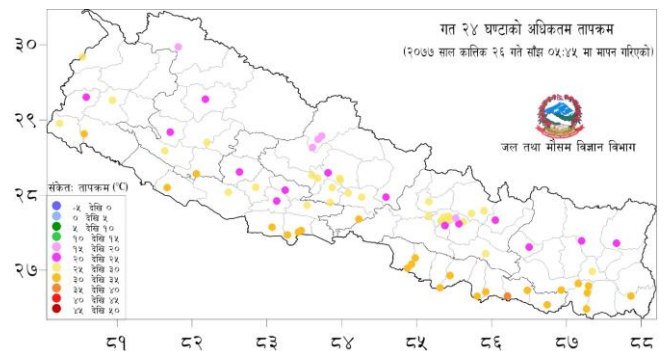
नक्सा २: कार्तिक २५ गते साँझ ०५:४५ बजे देखि कार्तिक २६ गते साँझ ०५:४५ सम्मको २४ घण्टाको अधिकतम तापक्रम
