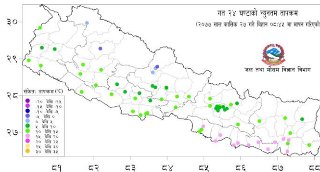
नक्सा १: कार्तिक २६ गते बिहान ०८:४५ बजे देखि कार्तिक २७ गते ०८:४५ बजे सम्मको २४ घण्टाको न्यूनतम तापक्रम
