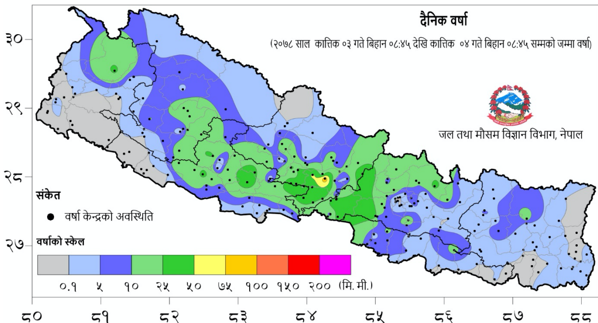
नक्सा १: कात्तिक ०३ गते बिहान ०८:४५ बजे देखि कात्तिक ०४ गते बिहान ०८:४५ बजे सम्मको २४ घण्टाको वर्षा (मि. मी.)
